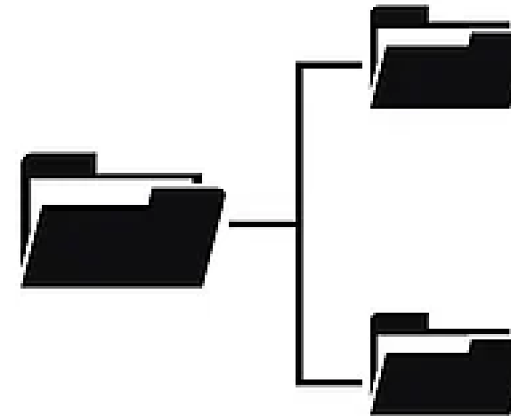
Ordnerstruktur
